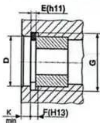
حلقة مرنة للأجواف NF E 22 -165
