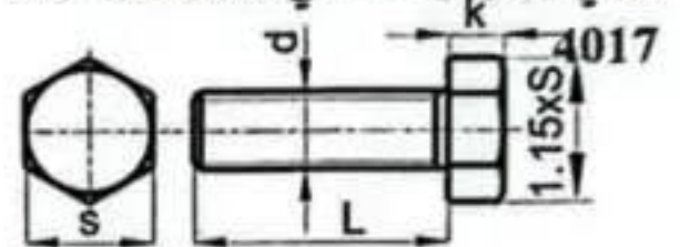
برغي ذو رأس سداسي NF EN ISO
