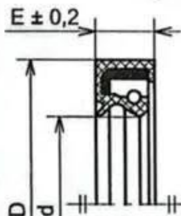
فاصل كتامة ذو شفتين نوع AS
