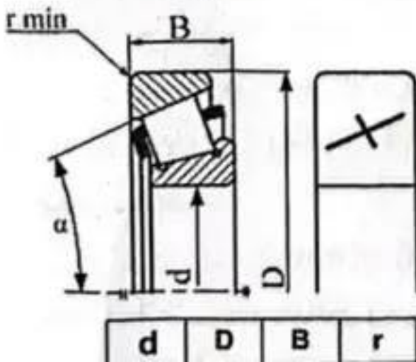
مدحرجة ذات الدحارج المخروطية
