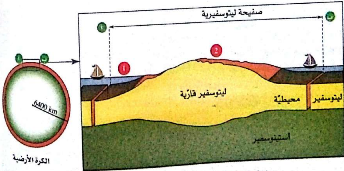
مقطع تخطيطي للصفحة الإفريقية
