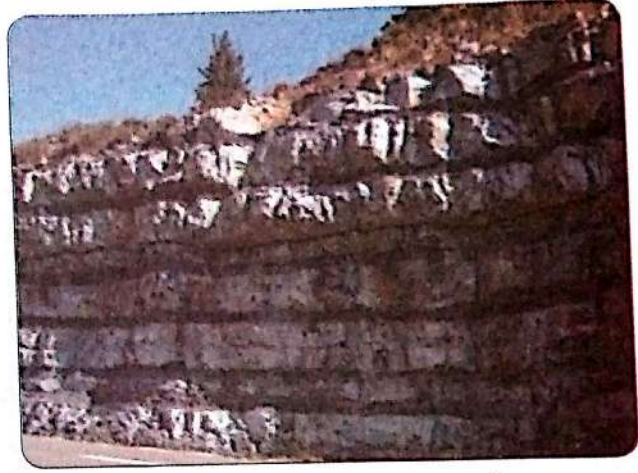
صخور ترسّبت على مدار زمن جيولوجي طويل.
