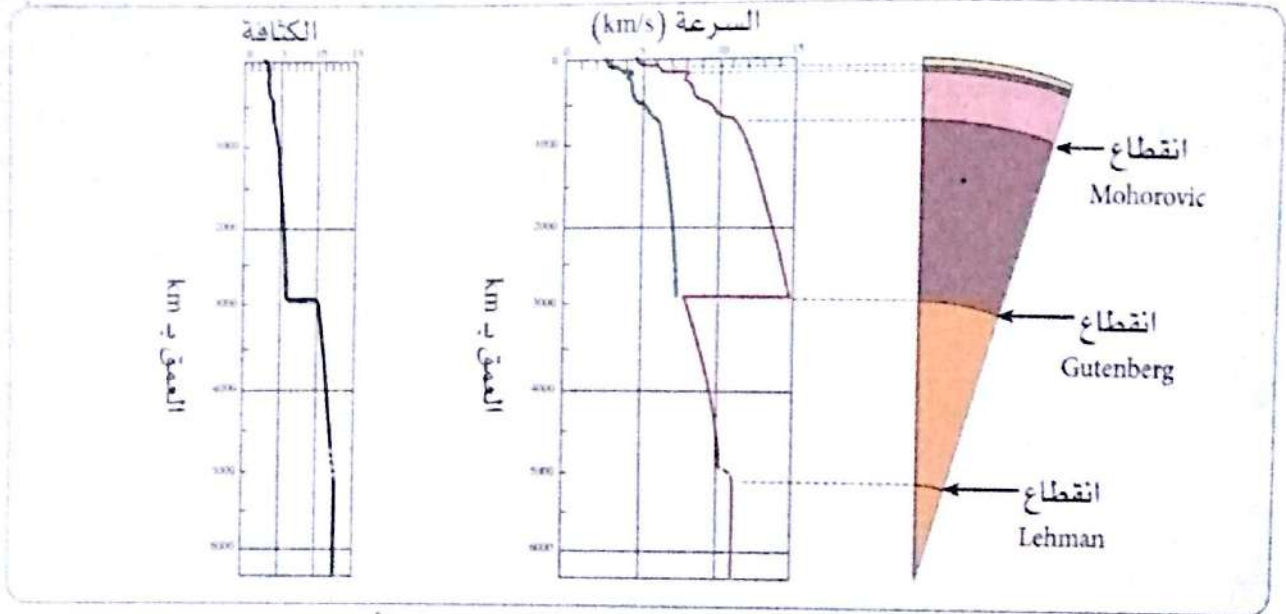
انتشار الموجات الزلزالية في المناطق العميقة للأرض
