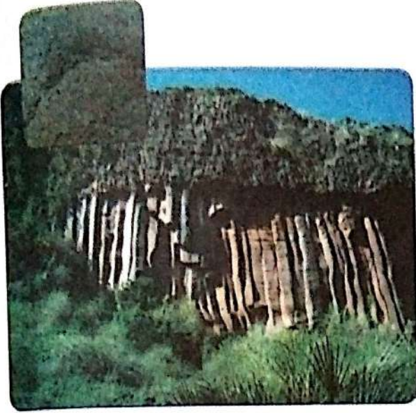
منظر بازلتى (تادمايت) : لونه داكن يميل إلى السواد، ذو حبيبات معدنية صغيرة ينتج عن الثوران البركاني (للافا تحت الماء).
