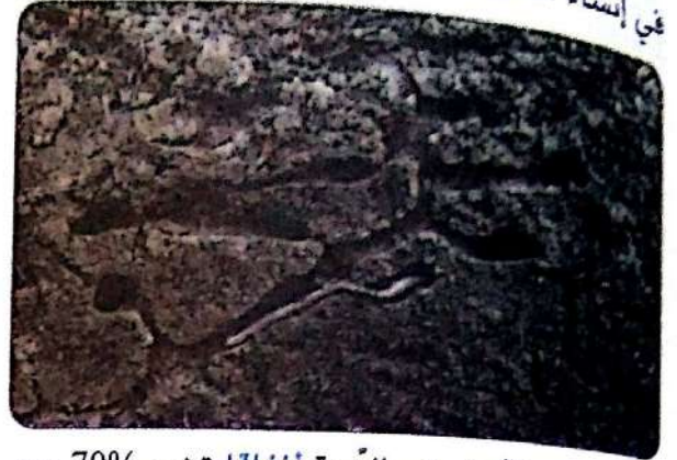
تحفر ديدان الأرض في التربة أنفاقا تضم 70% من الهواء الموجود في التربة، كما تخزن فيها الأوراق الميتة وتفتتها.
