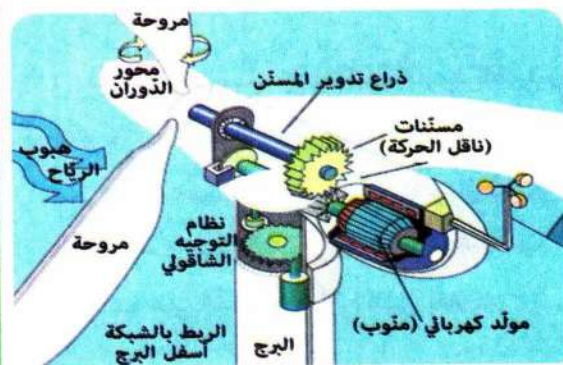
تركيبة توليد الطاقة الكهربائية من طاقة الرياح
