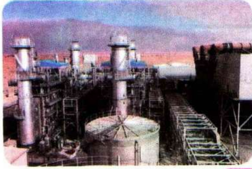
ولايه 7 المحطة الهجينة لإنتاج الطاقة الكهربائية بحاسي الرمل
