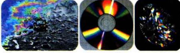
بقعة زيت على طريق مبللة
