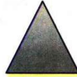
الموشور الأوّل
