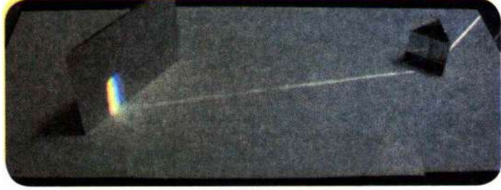
تحليل الضوء الأبيض بموشور
