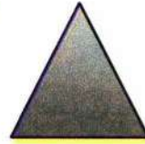
الموشور الثالث
