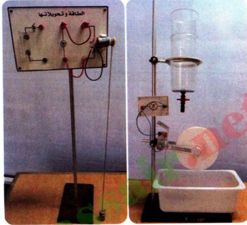
التركيب التجريبي لتوهج مصباح بواسطة تدفق الماء (يمين)، وبواسطة سقوط حجر (يسار)
