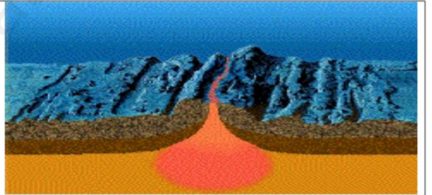
السند 02: البنية الجيولوجية المسؤولة عن زحزة القارات
