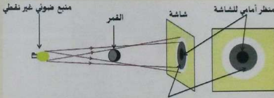
مخطط التركيب التجريبي
