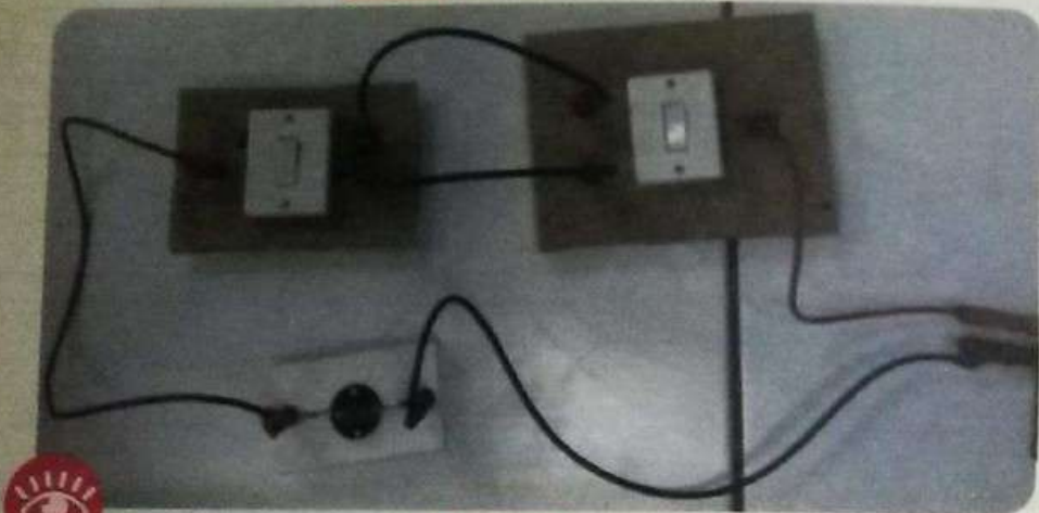
تحقيق الدائرة ذهاب - إياب
