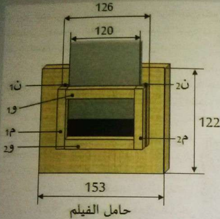
تحويل الحجرة المظلمة إلى آلة تصوير
