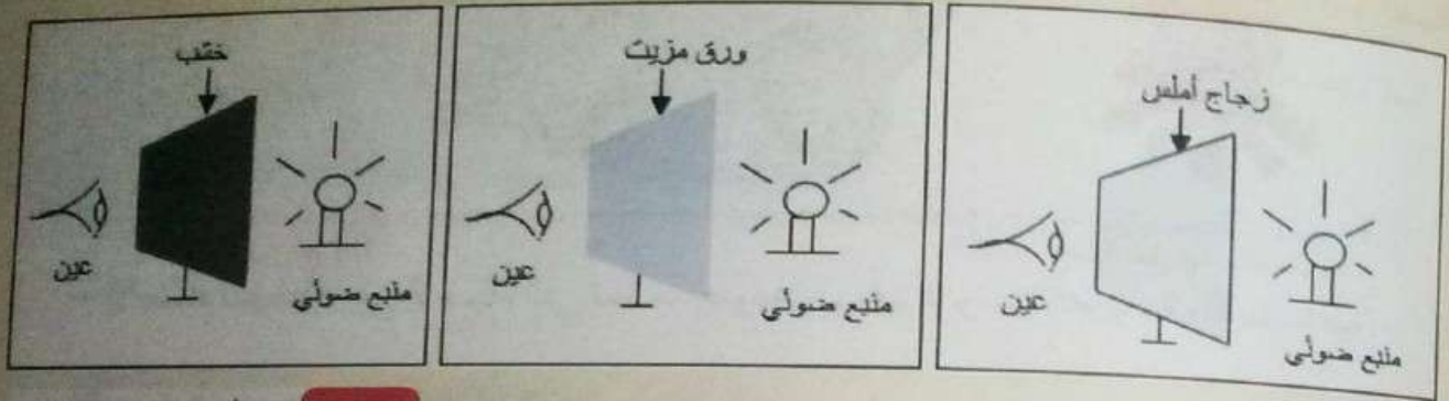
الأوساط الضوئية
