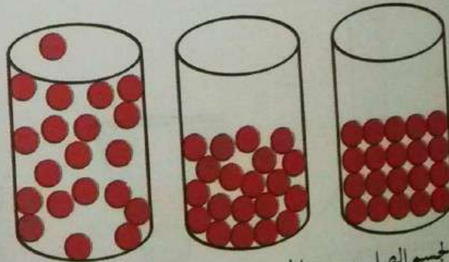
الجسم الغازي
