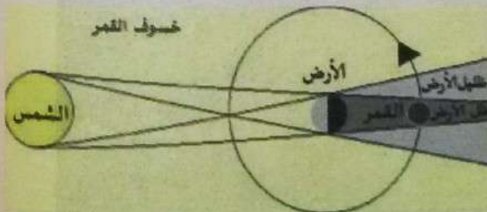
ظاهرة حدوث خسوف القمر
