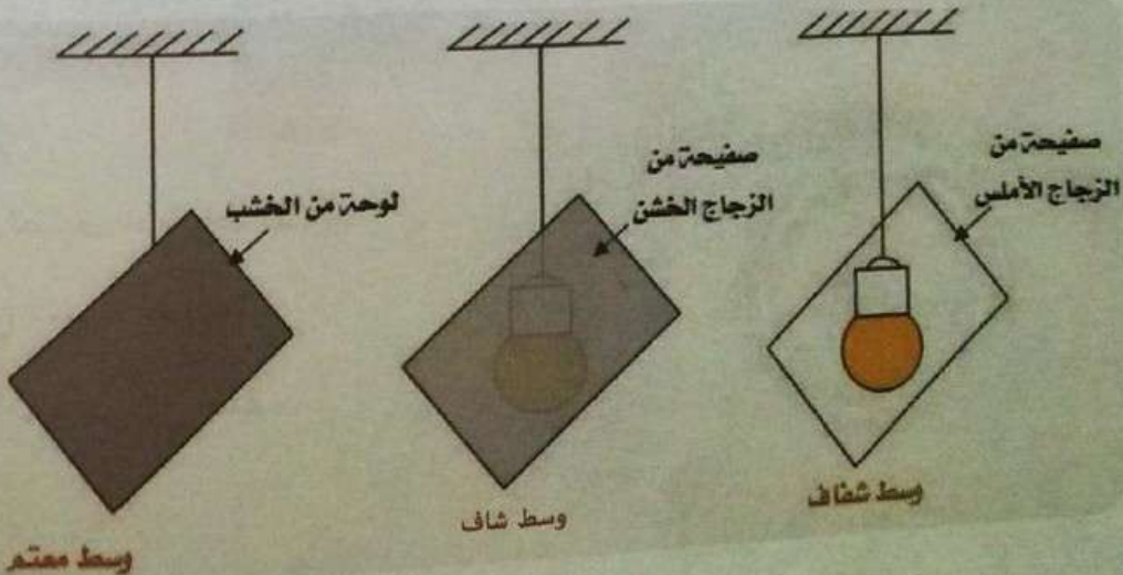
الأوساط الضوئية
