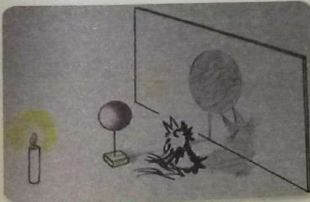
تشكّل الظل
