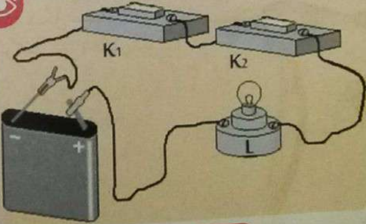
ربط القاطعتين على التسلسل
