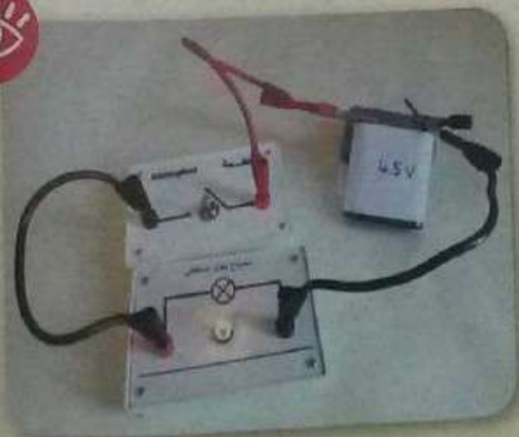
وثيقة 2 تركيب الدائرة
