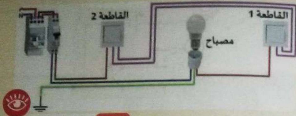
الدائرة ذهاب - إياب
