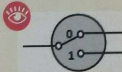
وثيقة 5 قاطعة مزدوجة
