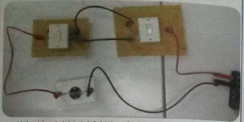
تركيب القاطعة في الدارة ذهاب- إياب في المخبر
