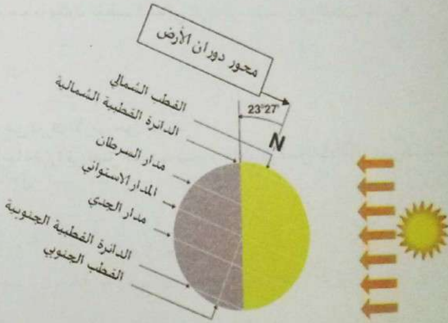
منحنى أشعة الشمس على الأرض في فصل الصيف
