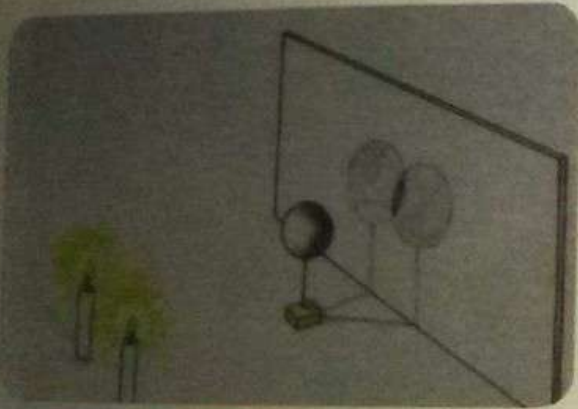
وثيقة 23 تشكل الظليل
