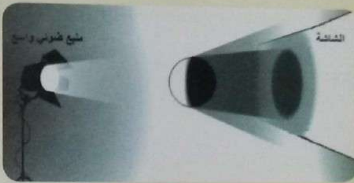
التركيب التجريبي
