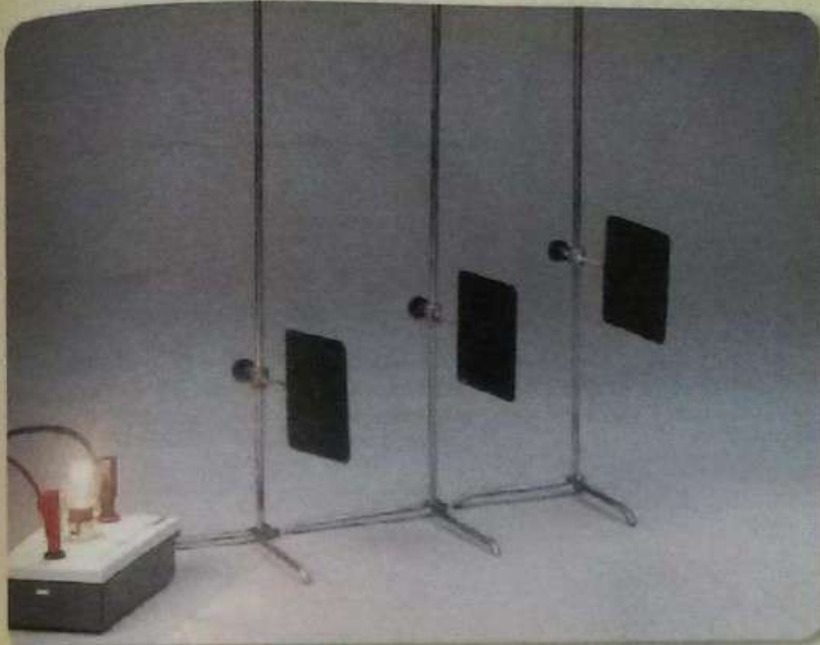
التركيب التجريبي
