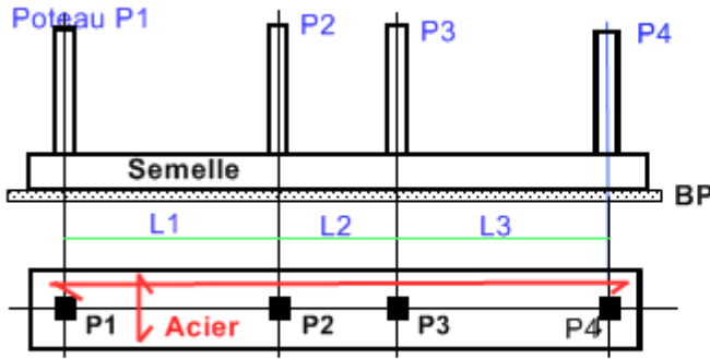
أساس مستمر تحت أعمدة
