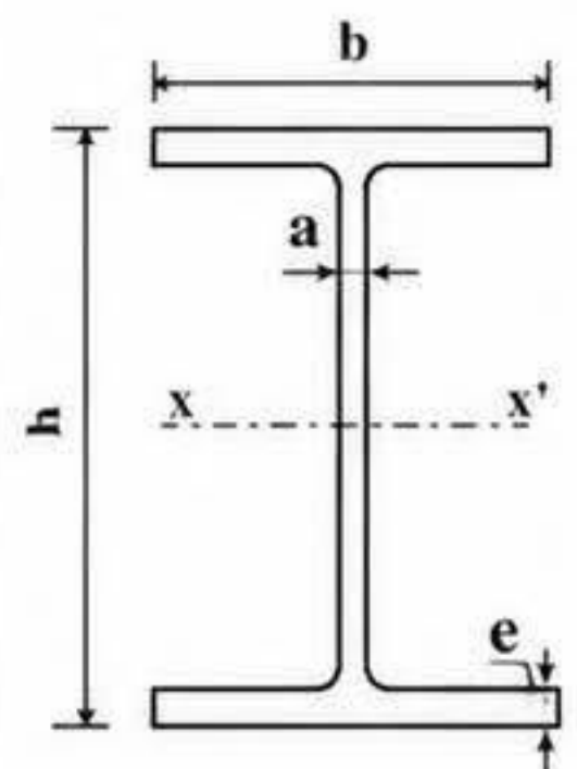
المقطع العرضي لمجنب IPE
